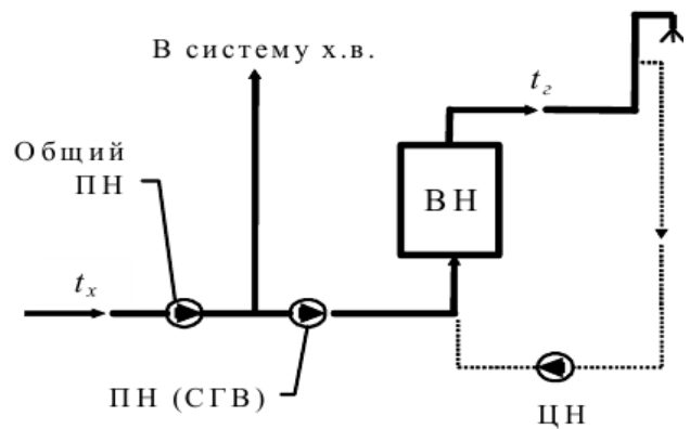
б) с общей повысительной установкой и дополнительным циркуляционным насосом СГВ
