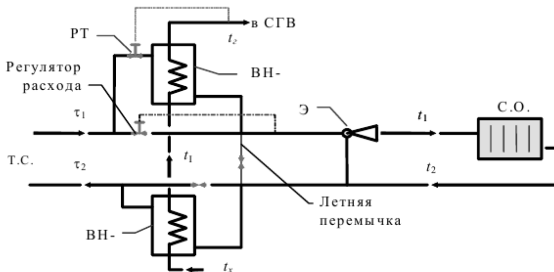
Рисунок 3.6. Двухступенчатая последовательная схема подключения водонагревателей ГВ к водяной тепловой сети
