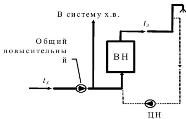
а) с общей повысительной установкой
