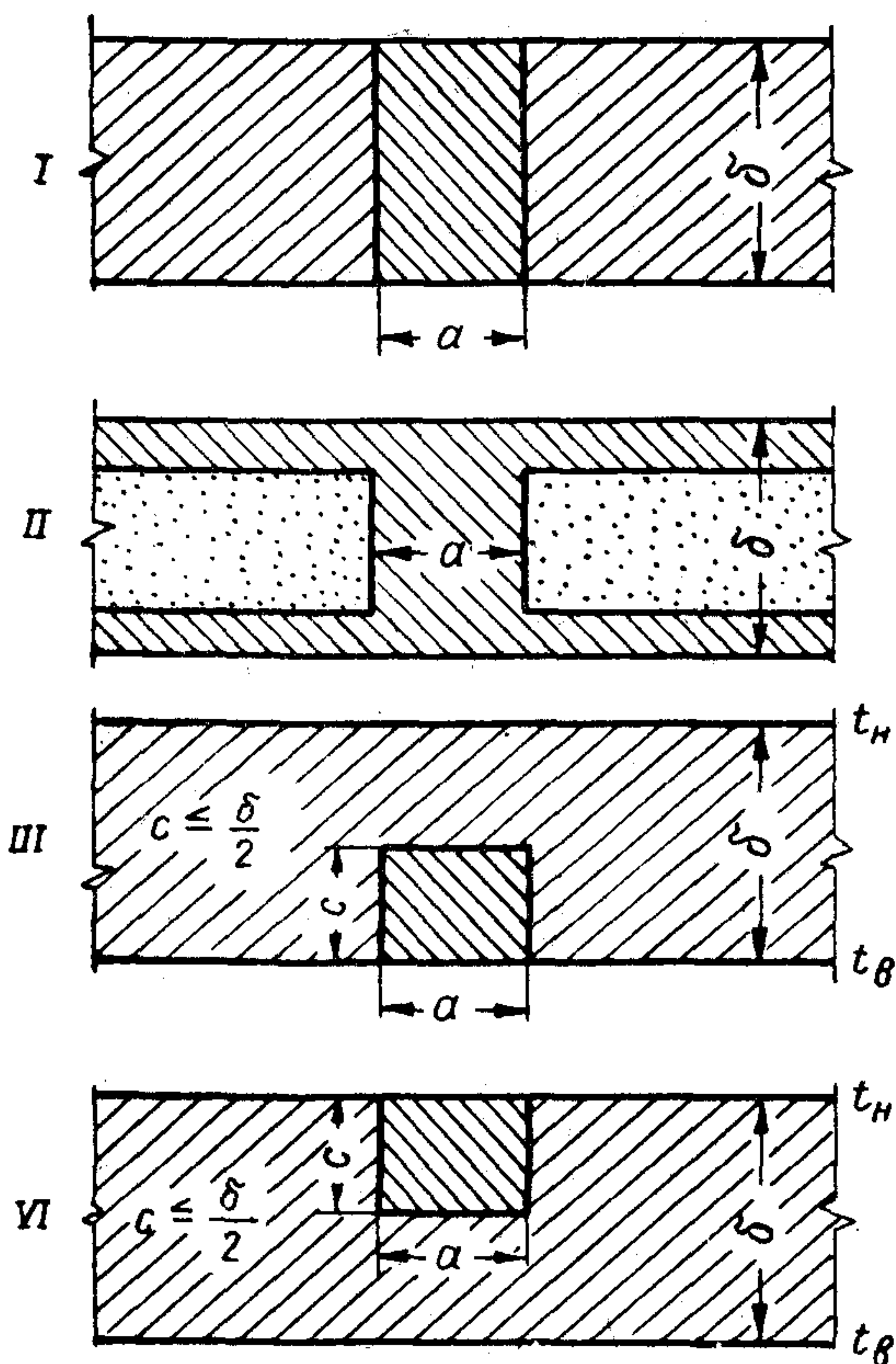
Рис. 2. Схемы теплопроводных включений в ограждающих конструкциях
