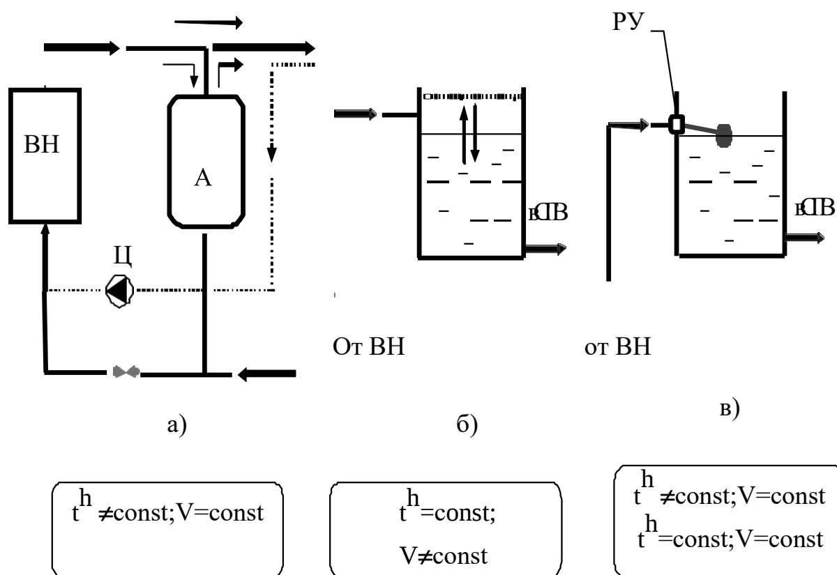
Рисунок 5.5. Варианты организации режимов работы баков-аккумуляторов: а) нижнего закрытого; б) открытого без регулятора уровня; в) открытого с регулятором уровня
