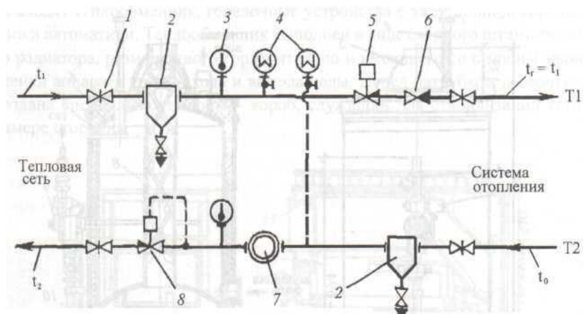
Рисунок 7.9. Схема местного теплового пункта при независимом присоединении системы отопления к квартальным тепловым сетям: 1 - задвижка; 2 - грязевик; 3 - термометр; 4 - манометр; 5 - регулятор расхода; 6 - обратный клапан; 7 - тепломер; 8 - регулятор давления
