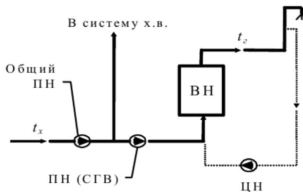
б) с общей повысительной установкой и дополнительным цирк. насосом СГВ
