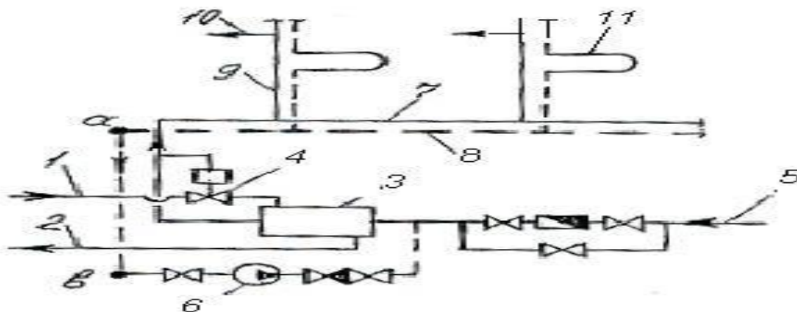
Рисунок 5.2. Схема горячего водоснабжения с нижней разводкой и принудительной циркуляцией. 1,2-трубопроводы тепловой сети; 3-водонагреватель;4-регулятор температуры; 5-водопроводная вода; 6-циркуляционный насос; 7-подающая линия; 8-циркуляционная линия; 9-разборный стояк; 10- к водоразборным приборам; 11- полотенцесушитель
