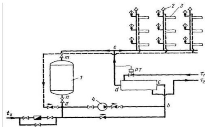
Рисунок 5.4. Схема горячего водоснабжения с нижним баком-аккумулятором. 1 – бак-аккумулятор; 2 – воздухоотводчик; 3 – полотенцесушитель; 4 – зарядочный насос.
