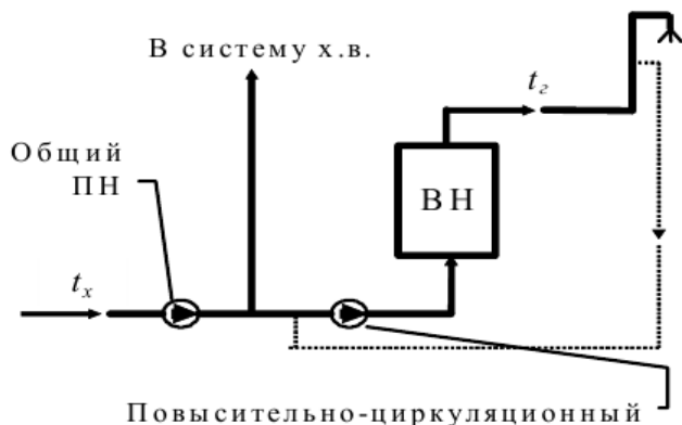
в) с повысительно-циркуляционным насосом СГВ
